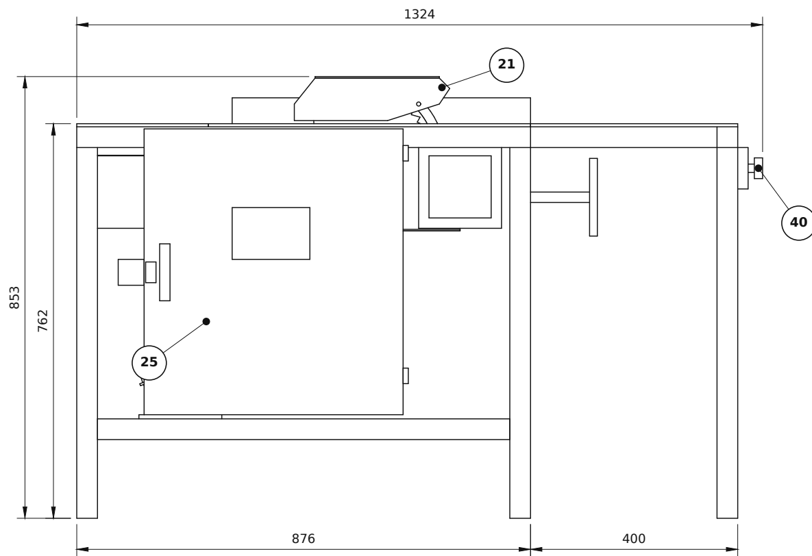
Vista Frontal Escala 1:10
