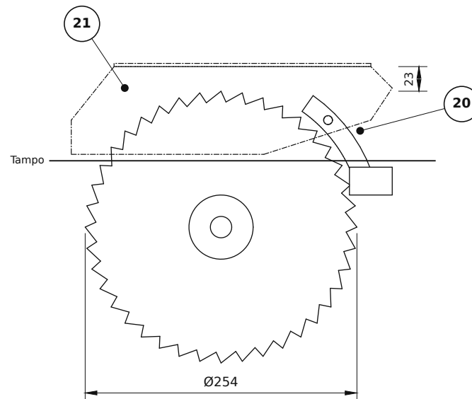
Detalhe A - Lâmina, Cutelo e Coifa Escala 1:5 · Coifa em Linha Fantasma
