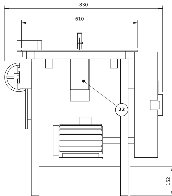
Vista Lateral Esquerda Escala 1:10
